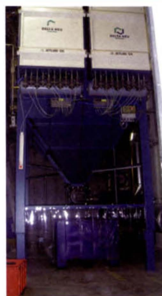
Un dépoussiéreur du type Jetline CH 80 Atox en acier peint installé à l'intérieur du bâtiment assure la filtration de l'air. Ce dépoussiéreur à poches filtrantes et à décolmatage par air comprimé permet d'obtenir un taux de rejet inférieur à 5 mg/m 3 . La mise en place sur la gaine de refoulement du ventilateur d'une sonde triboélectrique de type Dem 50 permet de contrôler en permanence le taux de poussières à la sortie du dépoussiéreur.
